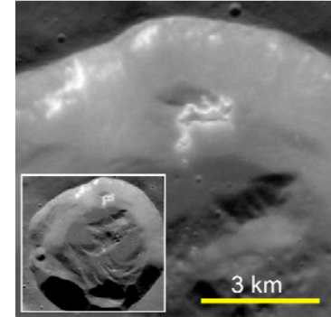
Pequeñas cavidades en la pared que le da la cara al sol en un cráter de 15 km. de diámetro. Exposición al severo ambiente del espacio en Mercurio es probablemente responsable por la formación de las cavidades.
