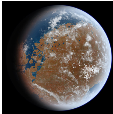
Un ambiente capaz de mantener agua en estado líquido en la historia temprana de Marte hubiera permitido la formación de carbonatos, y su subsiguiente entierro.
