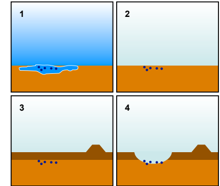
Posibles etapas en la formación, recubrimiento, y exposición de carbonatos en cráteres marcianos. Noten que otros procesos, como la actividad tectónica y fluvial, también son capaces de exponer rocas situadas debajo de la superficie.
