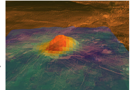
Observaciones infrarrojas de la nave espacial Venus Express superpuestas en la imagen de la ficha 1 muestran que Idunn Mons (rojo) tiene mayor emisividad térmica que sus alrededores (azul). Esto indica una diferencia de composición entre las dos regiones.
