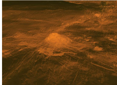
"Imagen" de radar y topográfica de Idunn Mons en Venus de la nave espacial Magellan. Se piensa que este volcán recientemente tuvo actividad. Las regiones oscuras son lisas y las regiones brillantes tienen alta rugosidad o pendientes empinadas. Las elevaciones han sido exageradas treinta veces.
