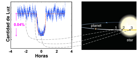
Las atenuaciones periódicas en la luz de la estrella son causadas por un planeta pasando por enfrente que posee un diámetro ~1.7 veces el de la Tierra.
