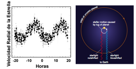
Los cambios en la longitud de onda medida de la luz de la estrella son causados por un planeta con masa ~5 veces la de la Tierra.
