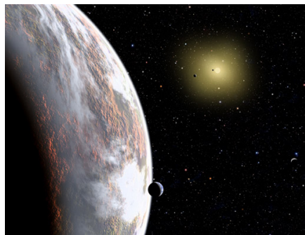
Identificación de mas exoplanetas rocosos ('Super-Tierras'), como los de esta interpretación artística, deben proseguir rápidamente gracias a telescopios espaciales dedicados por completo a esta labor, y a mejoras en las capacidades de detección desde la Tierra. Imagen cortesía de D. Aguilar, Harvard Smithsonian CfA.
